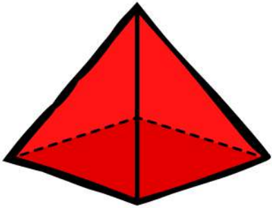
pyramid
